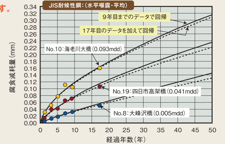
腐食減耗量の経年変化と式(1)の関係
