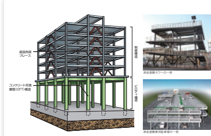
コンクリート充填鋼管柱の採用
