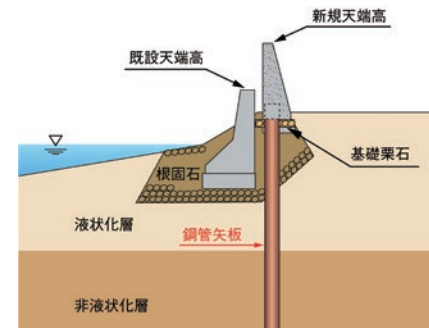
図-1 自立式
