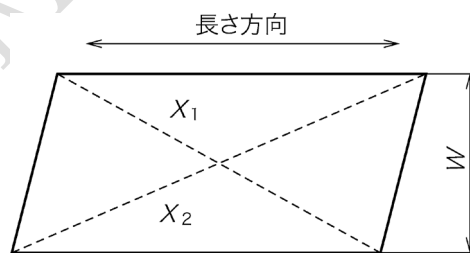
242 図 3—板及び波板の直角度（対角線を用いる方法）
