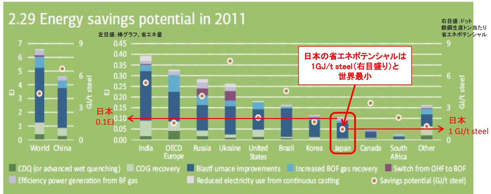
鉄鋼業の省エネポテンシャル国際比較(2011年時点)
